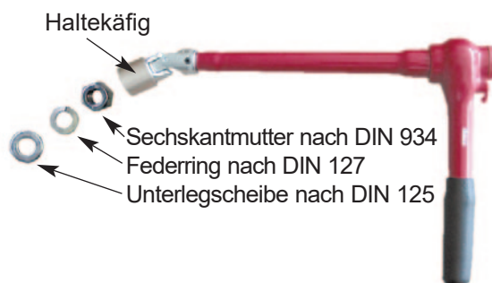
Abb. 10: Isoliersteckschlüssel mit Steckschlüssel-Einsatz SW 19 mit Mutter, Federring und Scheibe
