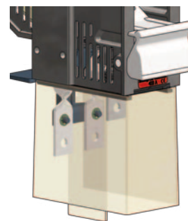
Abb. 7: Kabel-Abdeckhaube (L)
