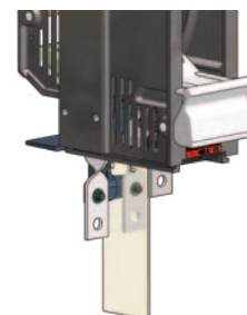
Abb. 14: Isolier-Trennplatte (K)
