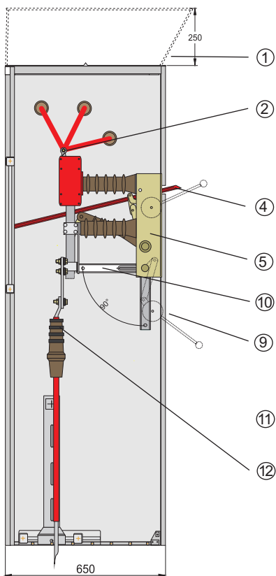
Bild 6: Seitenansicht Kabelfeld FK24-756519-27 mit Lasttrennschalter H27 EK
