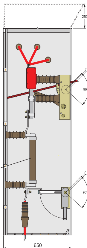
Bild 7: Seitenansicht Trafefeld FT24-756519-27 mit Lastschalter- Sicherungs-Kombination H27 SuT
