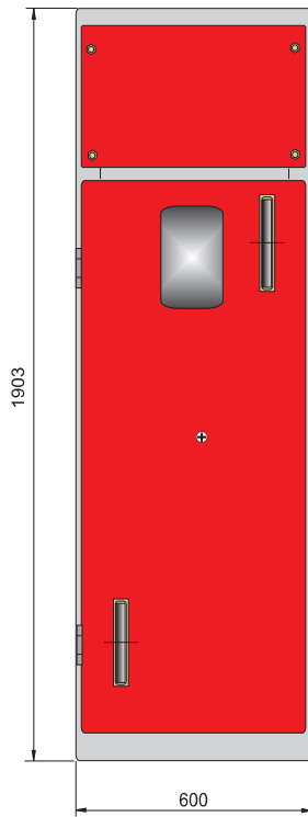
Bild 1: Frontansicht FT24-606519-27
