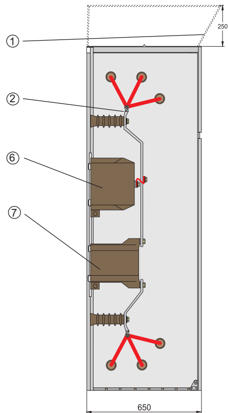
Bild 11: Seitenansicht Meßfeld FM24-907519 mit Schienenüberleitung sowie Strom- und Spannungswandlern
