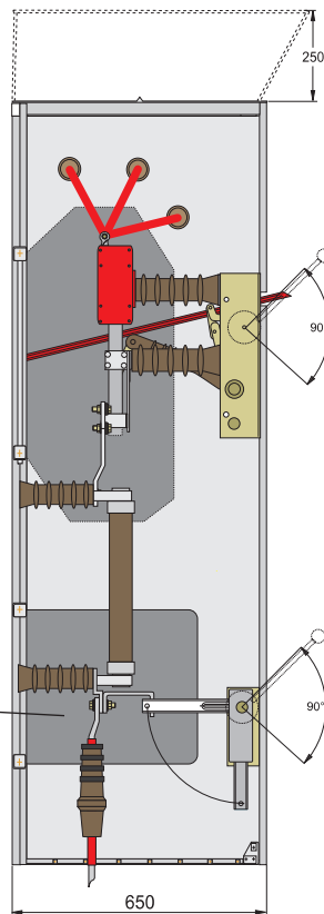
Bild 3: Seitenansicht Trafofeld FT24-606519-27 mit Lastschalter- Sicherungs-Kombination H27 SuT
