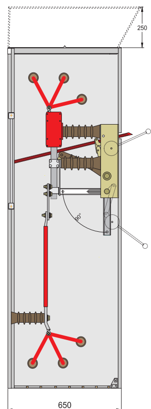
Bild 8: Seitenansicht Übergabefeld FÜ24-756519-27 mit Lasttrennschalter H27 EK
