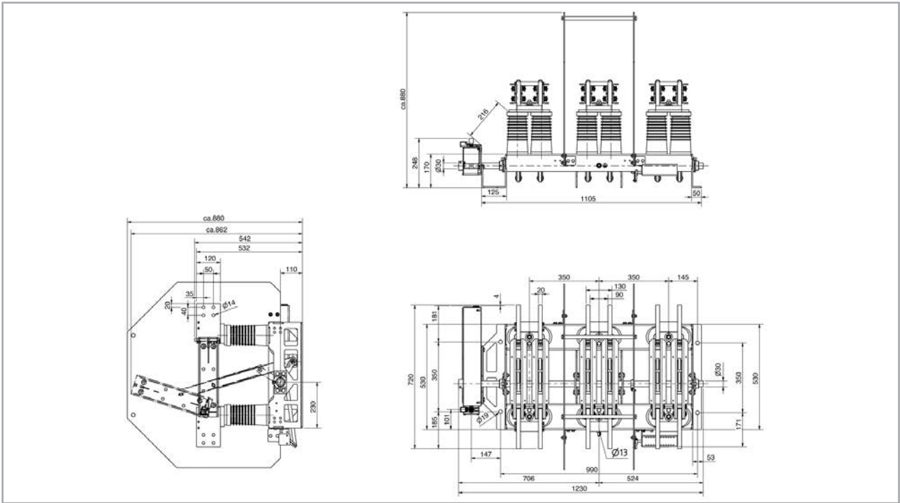
Zeichnung für ITr 24-6300-63 Hochkantanschluss / Zeichnungs-Nr. 117985
