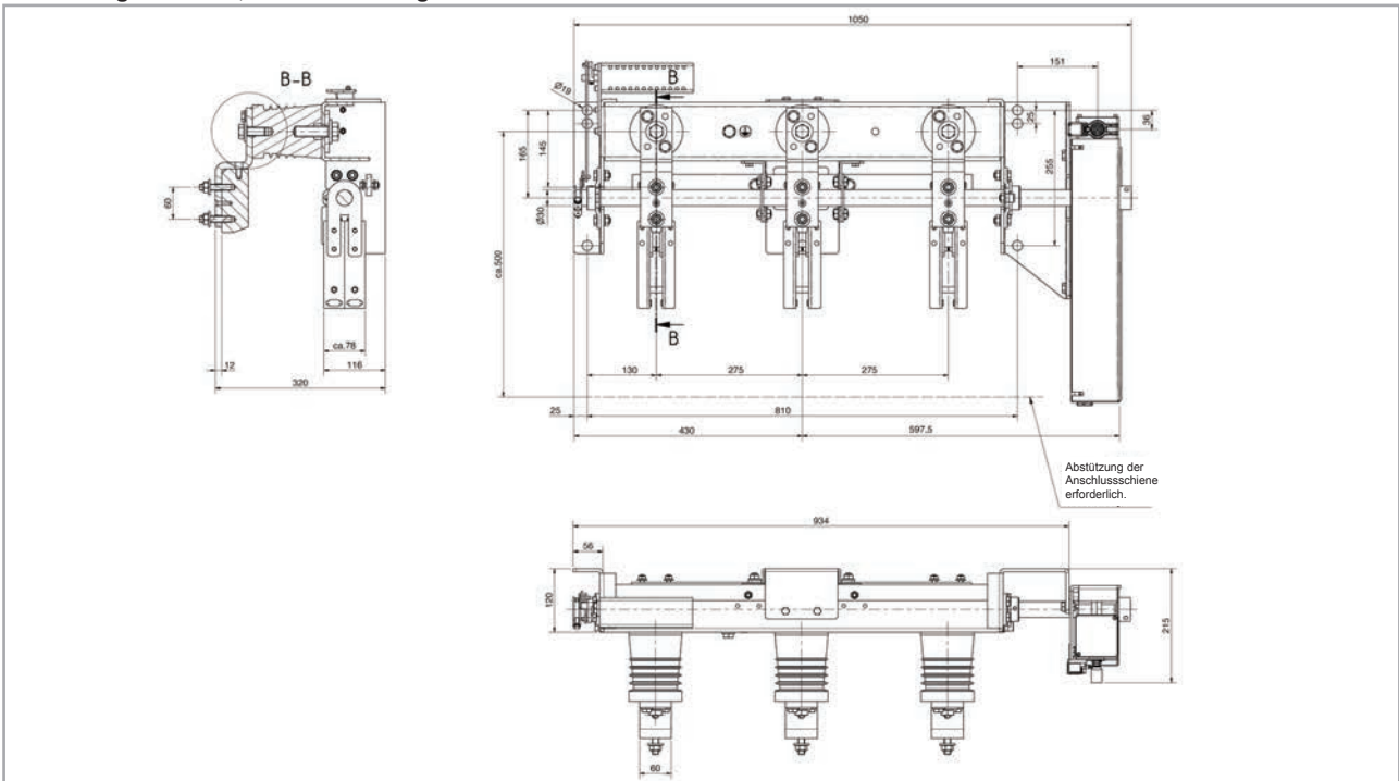
Zeichnung für ES 17,5-63 / Zeichnungs-Nr. 115712
