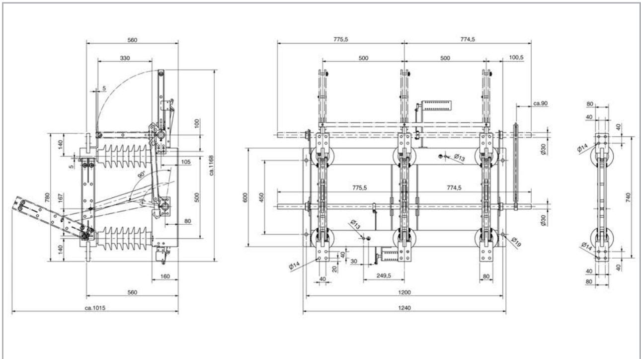
Zeichnung für ITr 38,5-2500-50, U r 40,5 kV / Zeichnungs-Nr. 108367
