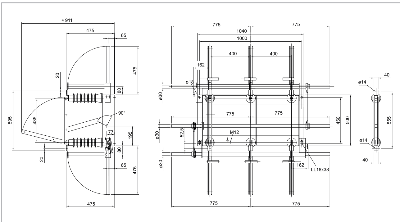
Abb.: ITr 38,5-1600-40
