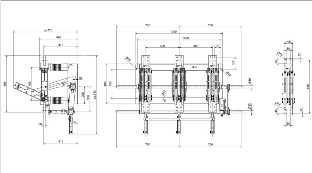
Zeichnung für ITr 24-4000-50 / Zeichnungs-Nr. 115630
