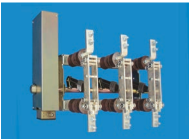
Abb.: ITr 12-1600-40
