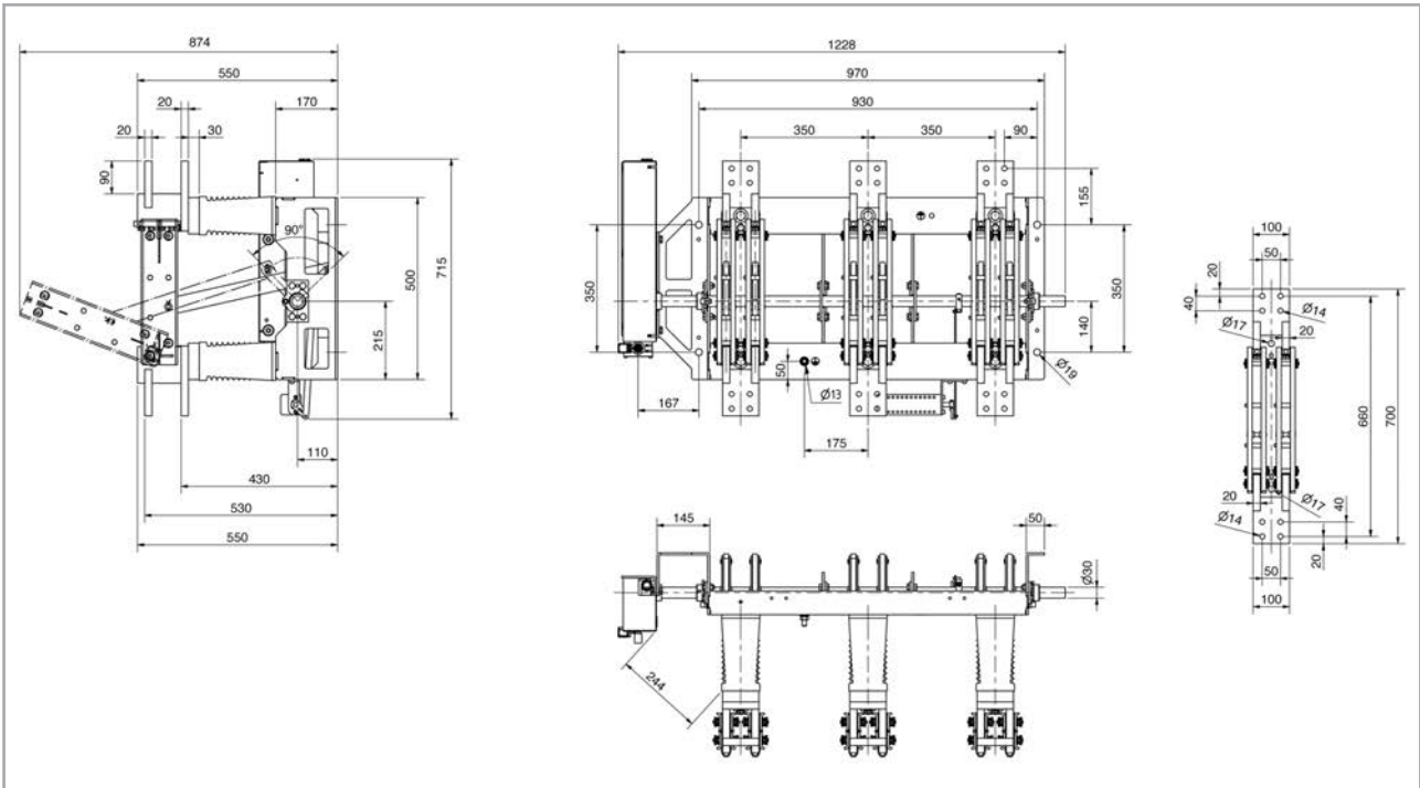
Zeichnung für ITr 24-6300-63 / Zeichnungs-Nr. 117673
