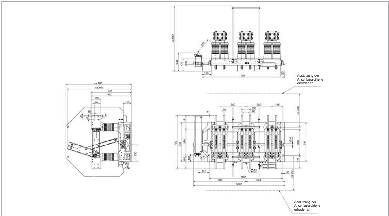
Zeichnung für ITr 24-6300-72 Hochkantanschluss / Zeichnungs-Nr. 117986
