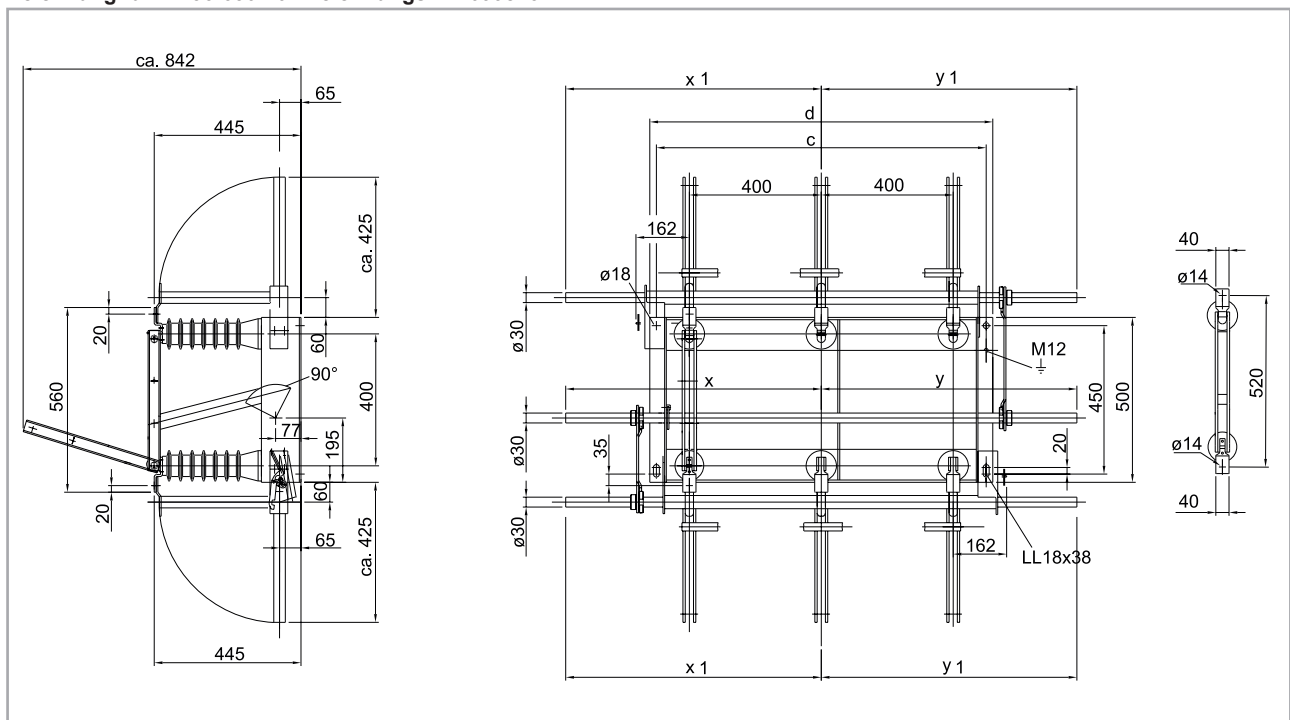
Abb.: ITr 36-1600-40
