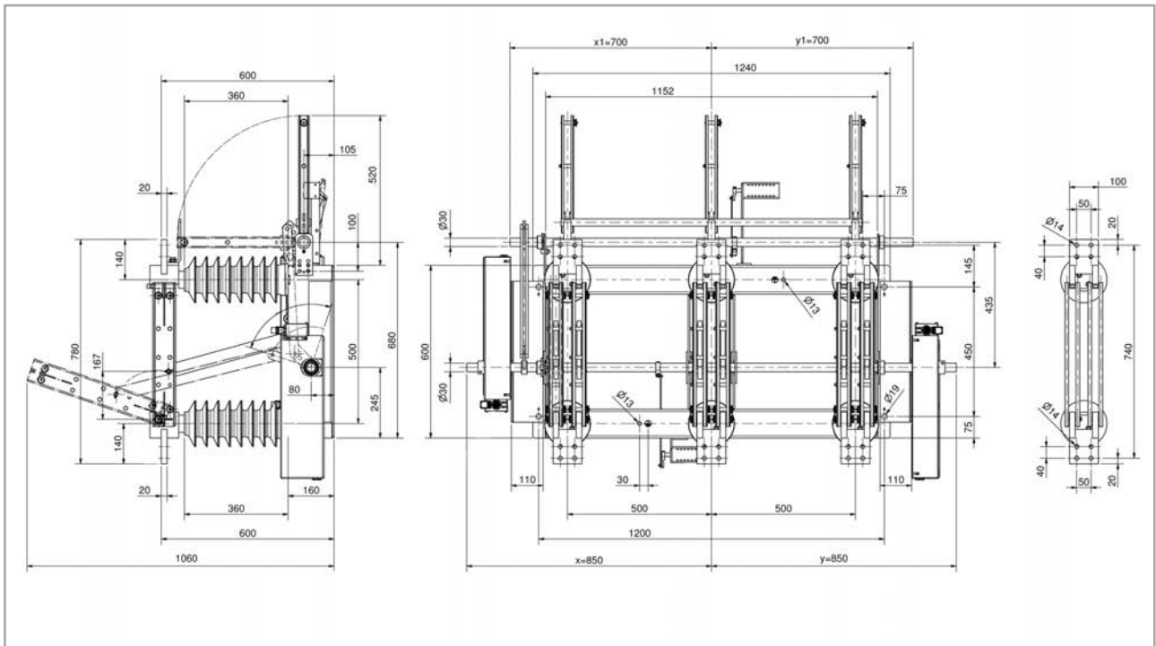
Zeichnung für ITr 36-4000-50, U r 40,5 kV / Zeichnungs-Nr. 113928
