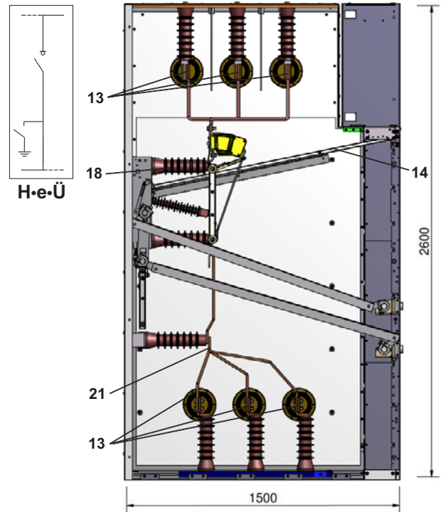
Abb. 16: PRO-AIR H-e-U, Ausführung Übergabefeld, 630 A Sammelschiene
