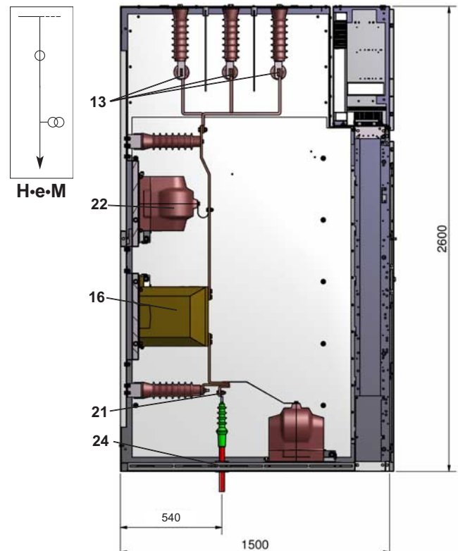
Abb. 18: PRO-AIR H-e-M, Ausführung Meßfeld, 630 A Sammelschiene
