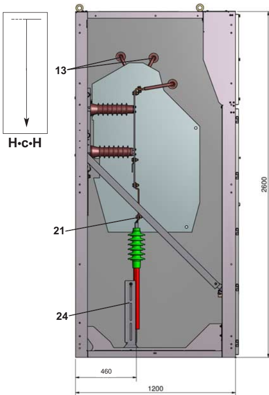
Abb. 11: PRO-AIR H-c-H, Ausführung Hochführungsfeld
