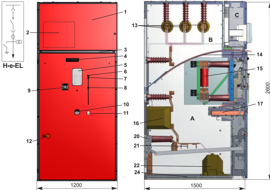
Abb. 23: PRO-AIR H•e•EL, Ausführung Einschubtechnik-Leistungsschaltfeld 31,5 kA, 2000 A Sammelschiene
