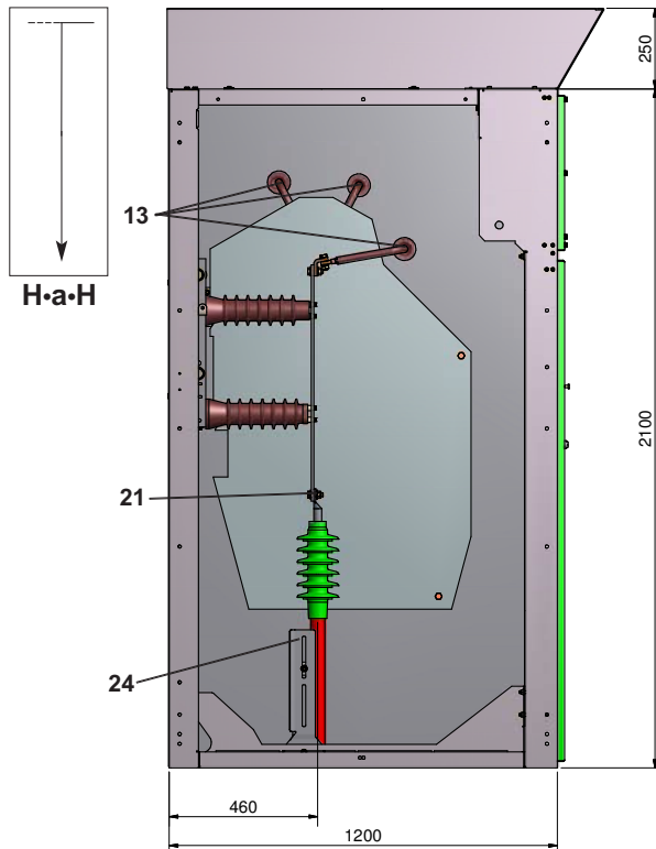
Abb. 6: PRO-AIR H-a-H, Ausführung Hochführungsfeld
