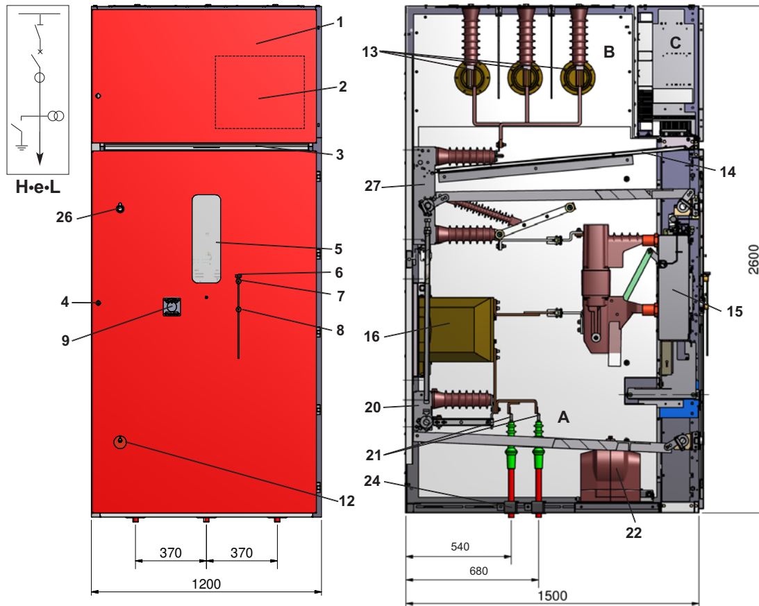
Abb. 19: PRO-AIR H•e•L, Ausführung Leistungsschalterfeld 20 kA (mobiler Festeinbau), 1250 A Sammelschiene
