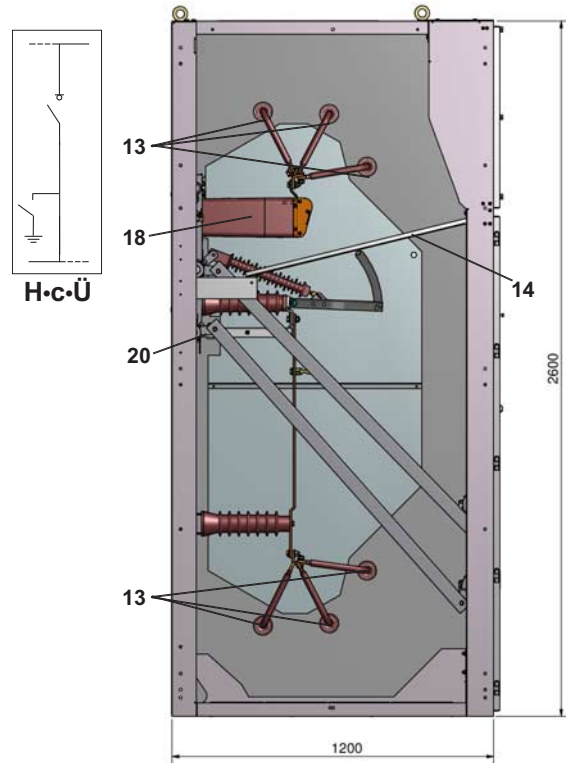
Abb. 10: PRO-AIR H-c-Ü, Ausführung Übergabefeld
