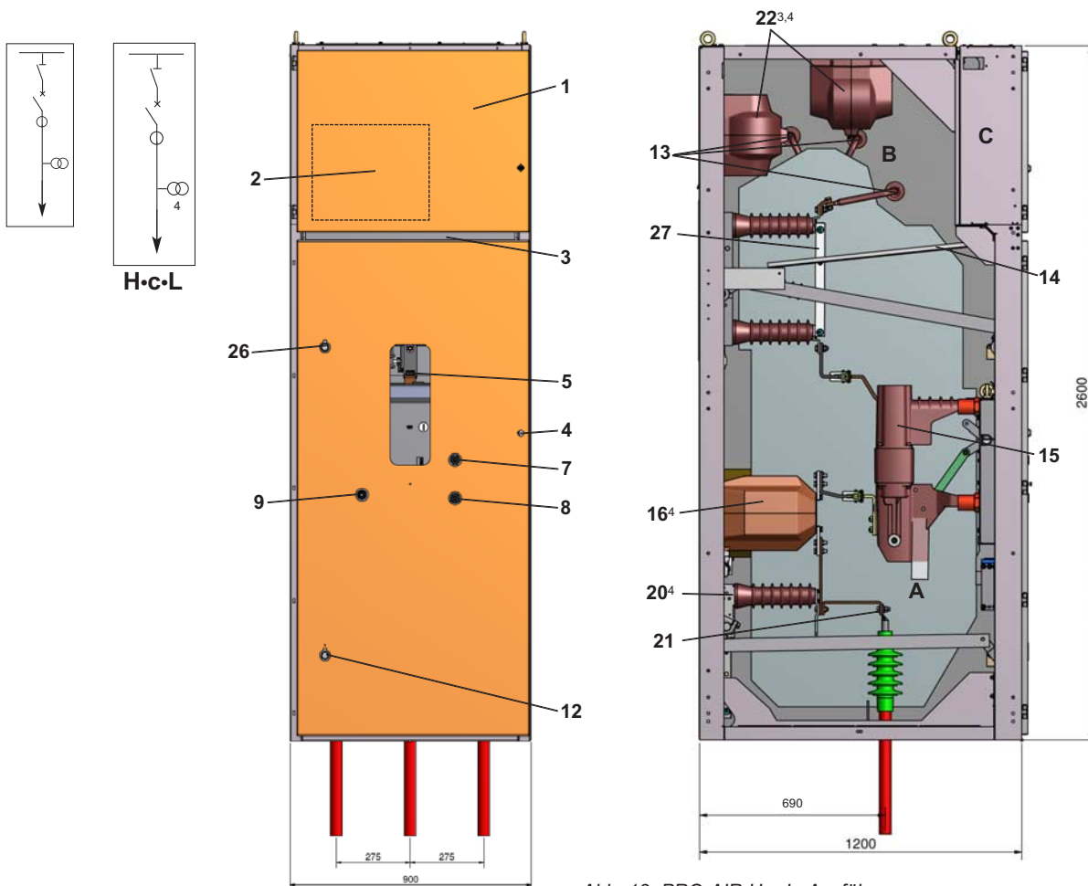
Abb. 13: PRO-AIR H•c•L, Ausführung Leistungsschalterfeld (mobiler Festeinbau)
