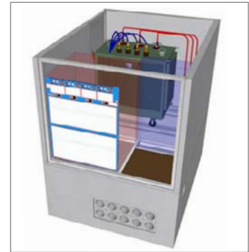
Abb.: oben Darstellung ECOS-C in nichtbegehbaren Station, unten nichtbegehbare Station
