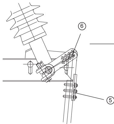
Kurbelstellung
