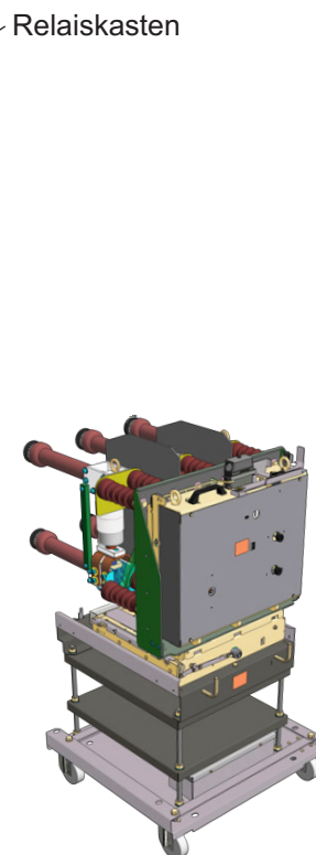
Typ E3K24-101624: Einspeiseschaltfeld mit Servicewagen, Leistungsschalter in Trennstellung
