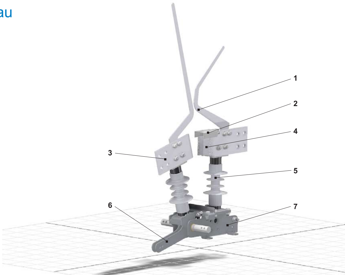
Abb. 2: OL-DC - LBS
